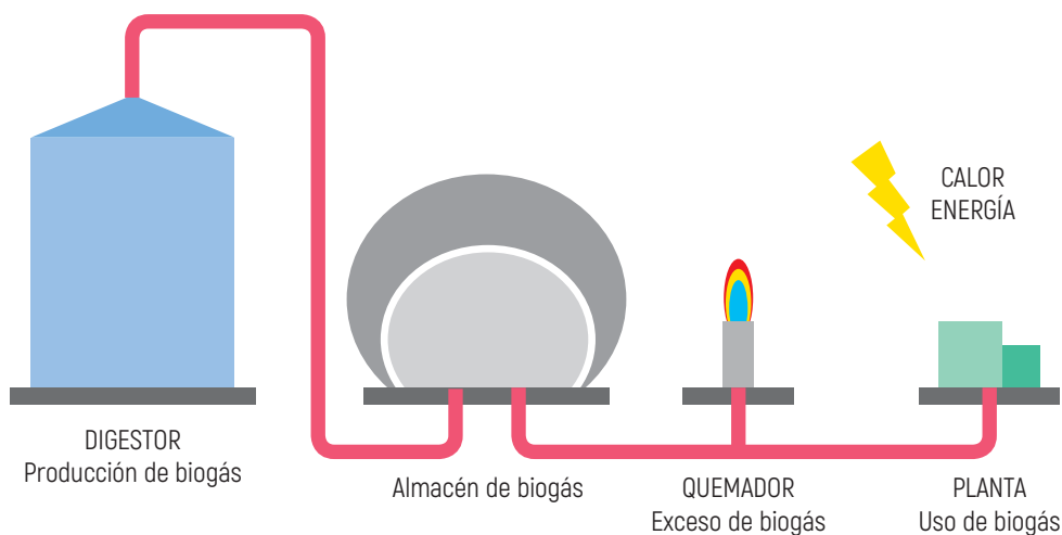
Ilustración 24. Esquema general de un sistema de digestión anaerobia
