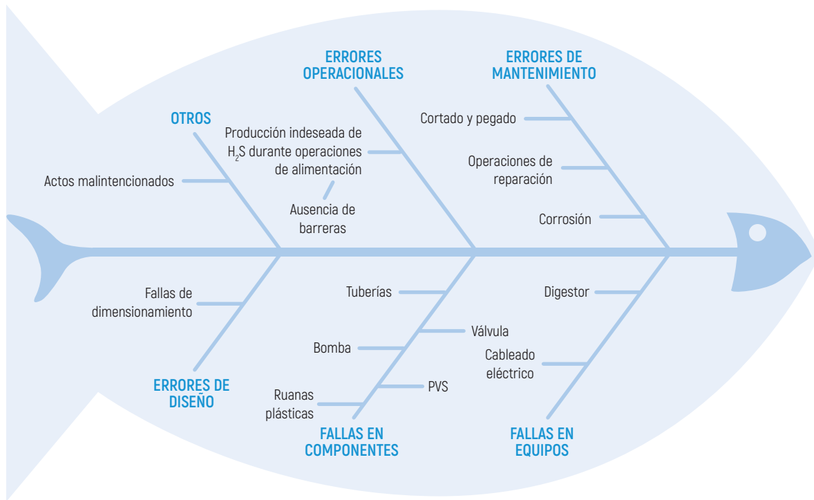
Ilustración 23. Diagrama de espina de pescado de las causas de accidentes en plantas de biogás.
