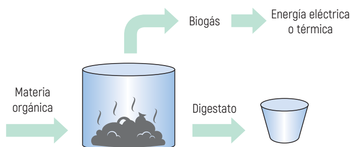
Ilustración 3. Esquema básico del proceso de digestión anaerobia.
