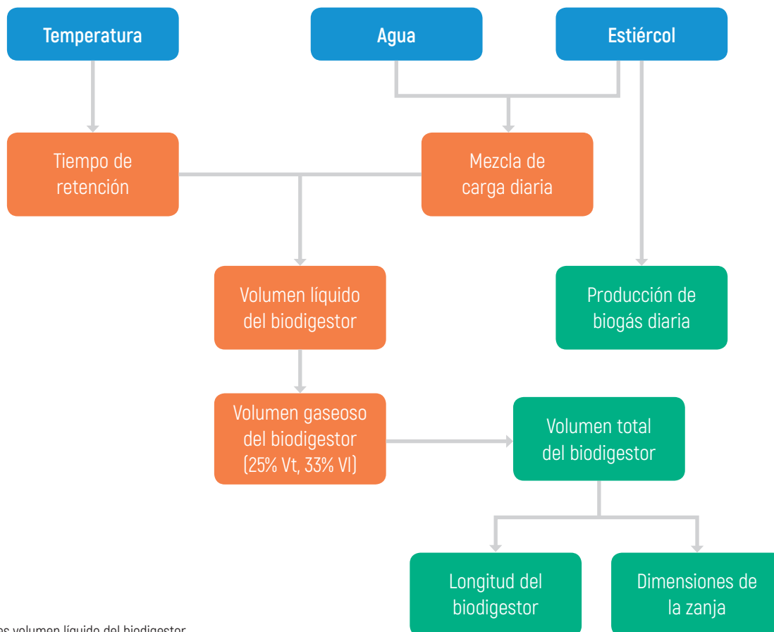
Ilustración 19. Esquematación de la metodología para el dimensionamiento de un biodigestor de flujo continuo
