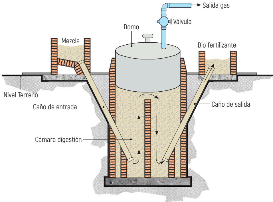
Ilustración 17. Biodigestor tipo hindú
