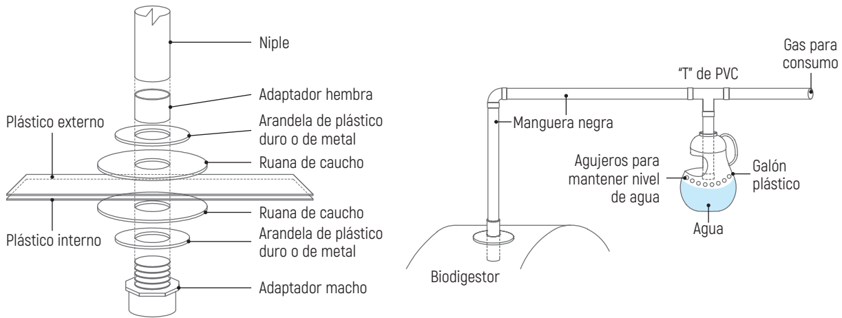
Ilustración 20. Instalación de salida del biogás y válvula de seguridad
