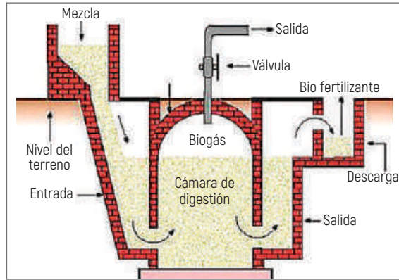
Ilustración 14. Biodigestor tipo hindú
