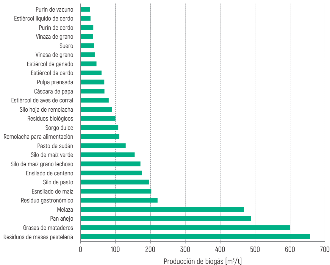
Ilustración 10. Rendimiento medio en biogás de diferentes materias primas
