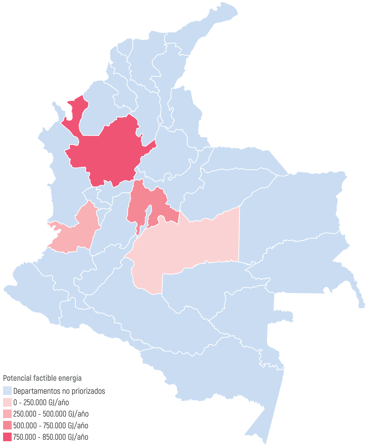
Ilustración 11. Potencial factible de generación de biogás a partir de porcínaza
