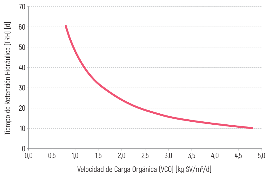
Ilustración 9. Correlación entre la tasa de carga orgánica y el tiempo de retención para la porcinaza
