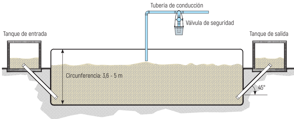
Ilustración 18. Biodigestor tipo Taiwán
