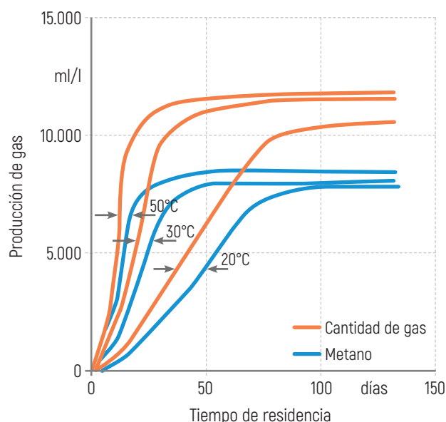
Ilustración 8. Temperaturas del proceso de digestión anaeróbica
