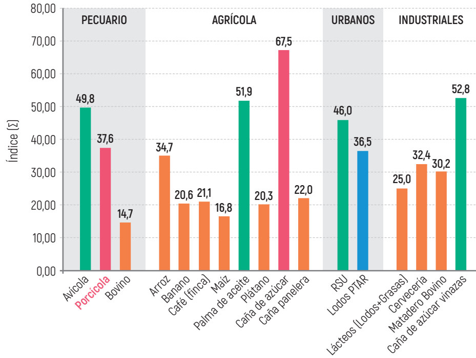
Ilustración 12. Biomásas residuales priorizadas para generación de biogás
