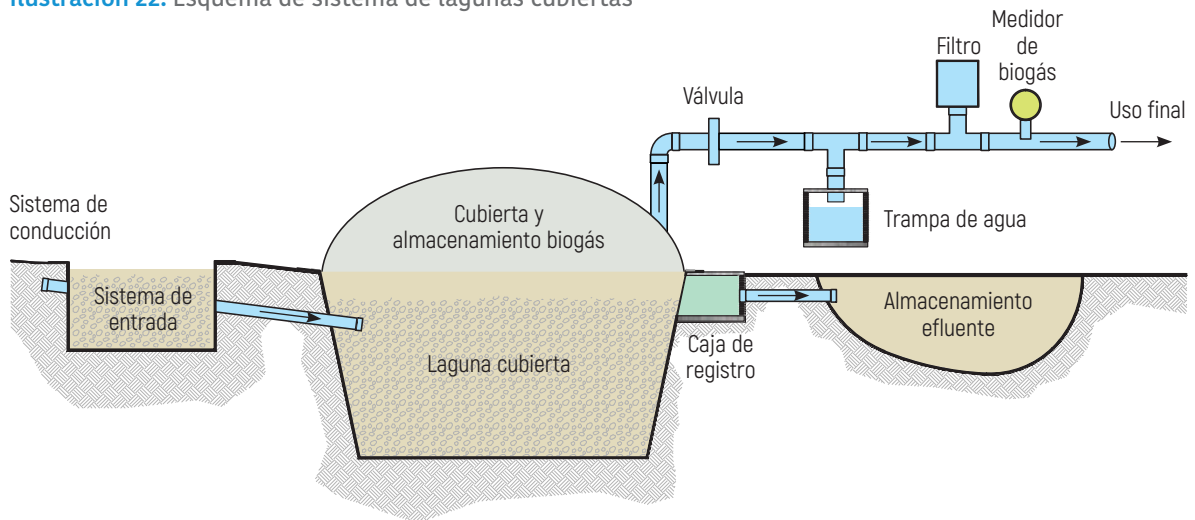
Ilustración 22. Esquema de sistema de lagunas cubiertas
