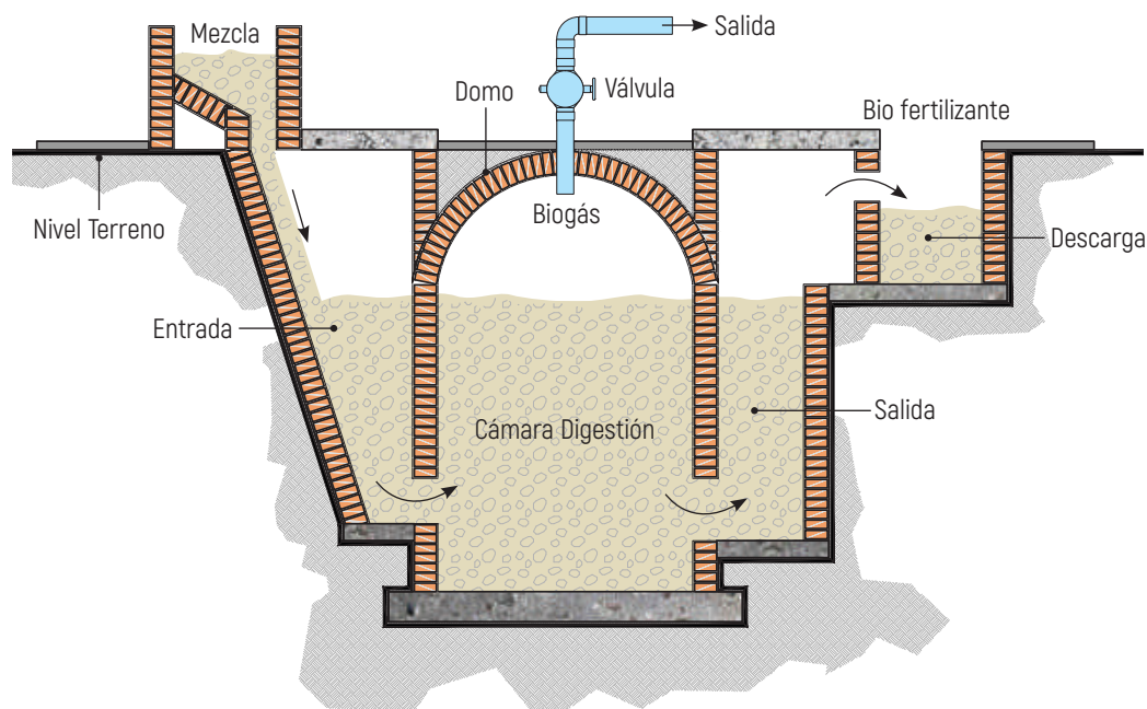
Ilustración 16. Biodigestor tipo chino
