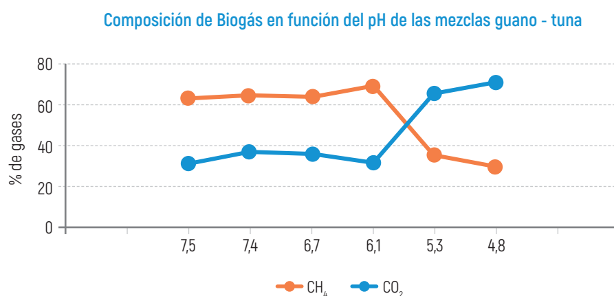
Ilustración 7. Variación en la composición del biogás en función del pH
